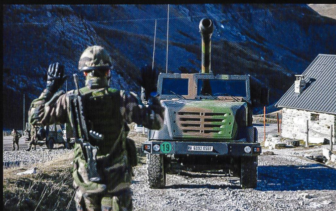
Plus de 77 Césars sont en service au sein de l'armée française. Le système pèse 19 tonnes et est monté sur un châssis Unimog qui confère un certain degré de protection à l'équipe durant les déplacements.
