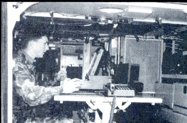
Char PCT de l'artillerie, avec les systèmes d conduite FARGO et INTAFF .
