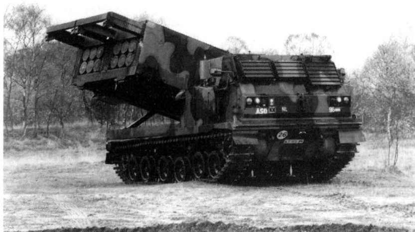
Lance-fusées multiples (Photo: MLRS International Corp.)
