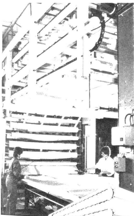
Paternoster à pont pour plus de 100 rouleaux de tissus avec motifs différents. Charge totale de 5 t. H 4,2 m. L 2,8 m. P 5,9 m.
