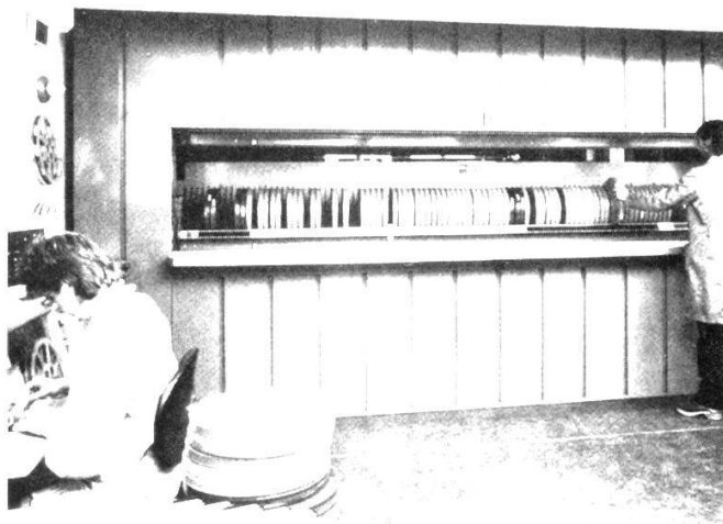
Paternoster horizontal à serpents pour bobines de films et cassettes vidéo de l'armée suisse. 40 nacelles.
