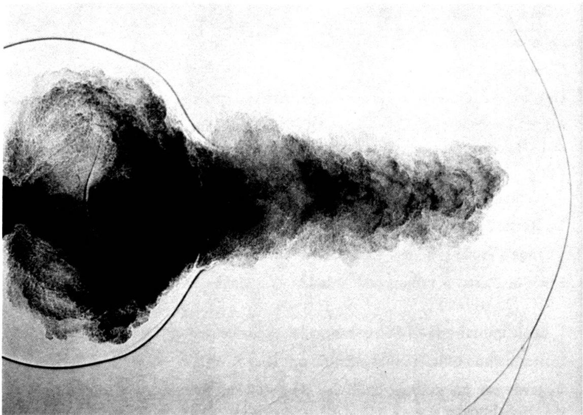
Image strioscopique d'une balle de pistolet quittant le canon, prise par le Groupement de l'armement en collaboration avec Polaroid.
