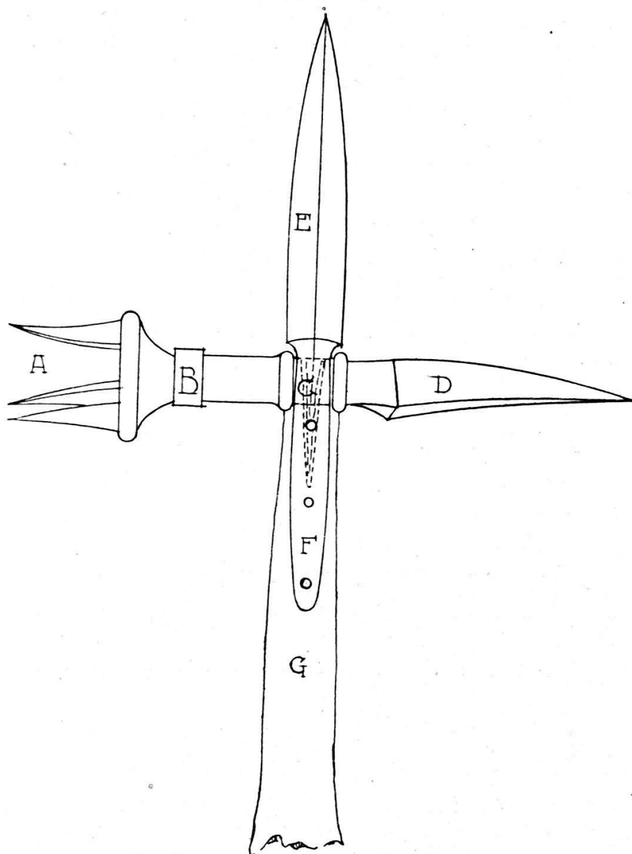
FIG. 2. — La masse d'arme reconstituée.
