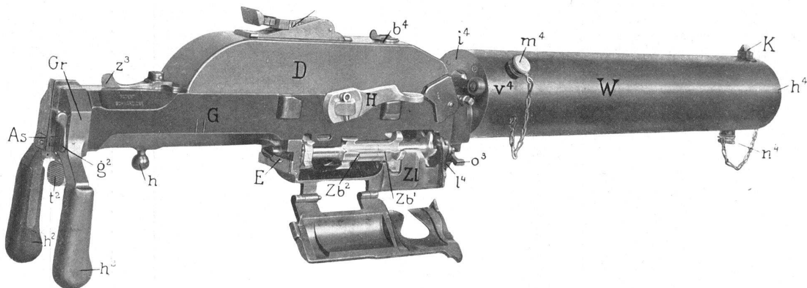
Mitrailleuse Schwarzlose, vue à droite, le support du distributeur étant ouvert.
