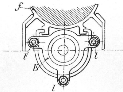
fig. 4 Vue arrière du berceau.
