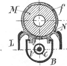
fig. 3 Coupe suivant f
