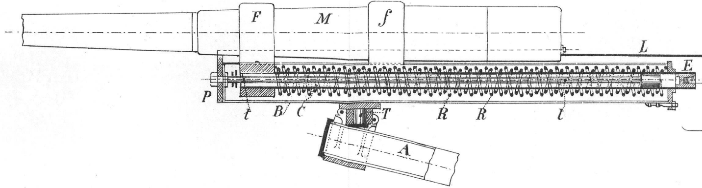
fig. 1. Bouche à feu et berceau.
