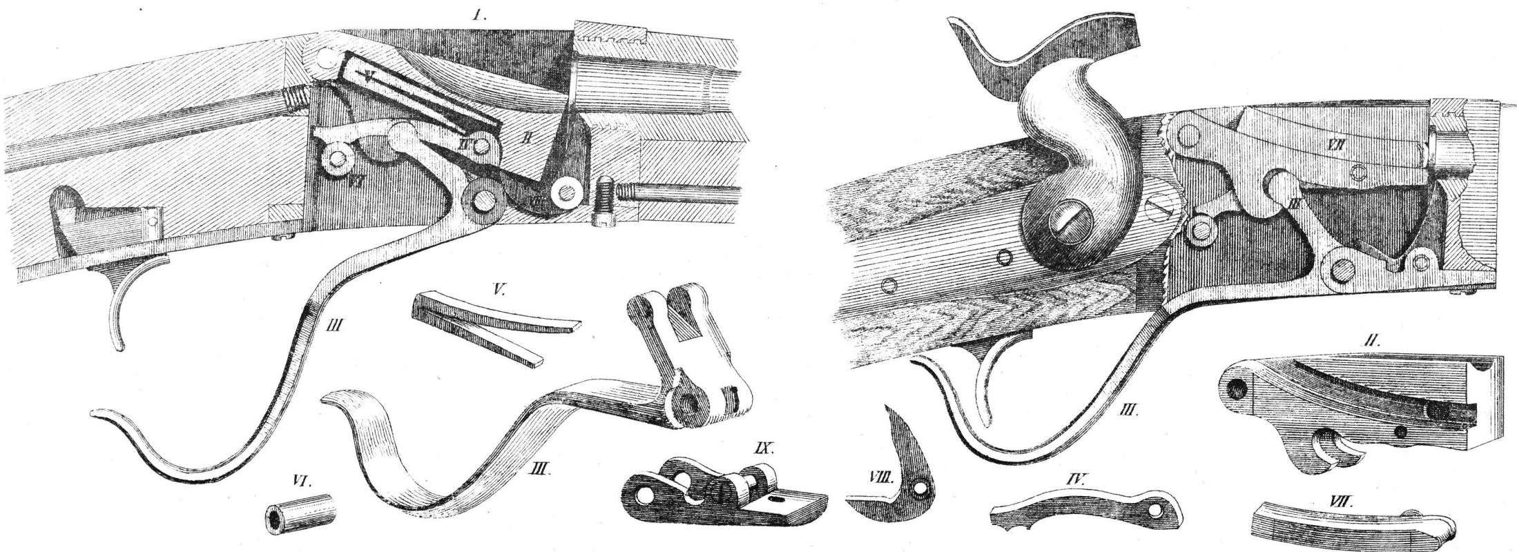
I. Boîte de Culasse. II. Obturateur. III. Pontet coude. IV. Pièce d'arrêt. V. Ressort d'arrêt. VI. Cylindre. VII. Broche. VIII. Extracteur. IX. Support de l'Extracteur.
