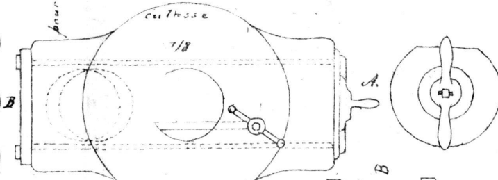
Coupe longitudinale de la culasse suivant A.B.
