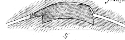
Profil de la rayure et de l'ancienne ailette du canon français de 30 Lb.
