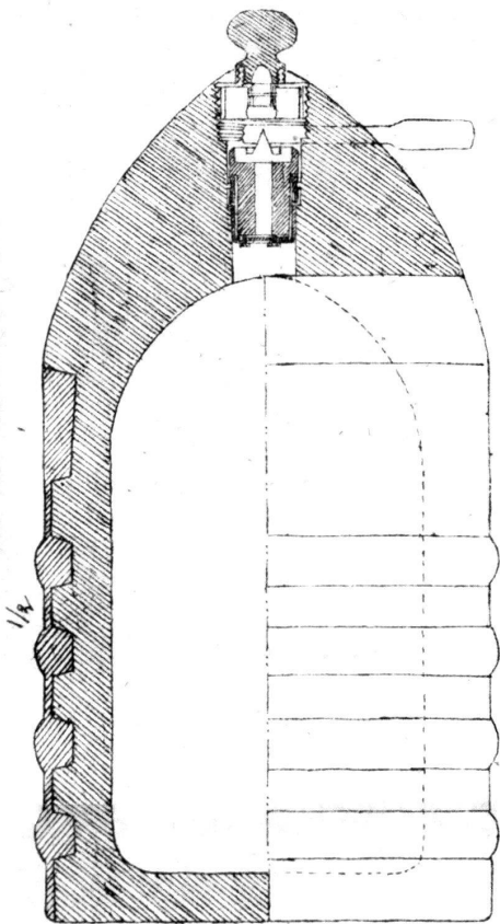
pour canons de 12 lb. avec anneau en cuivre.
