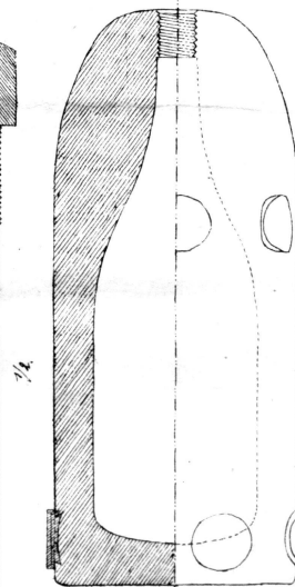
Obus pour canons de 30 Lb. \frac{1}{16}
