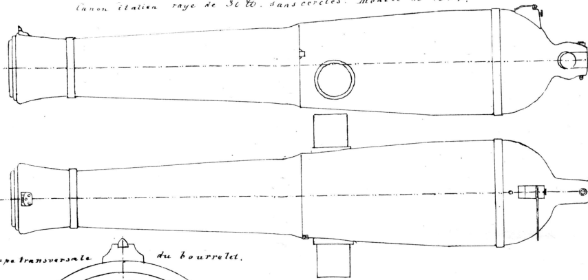
\frac{1}{8} Rayure rétrécie.
