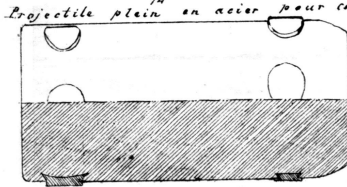
Projectile plein en acier pour canons de 30 Lb.
