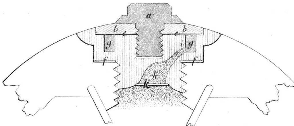
Coupe.
