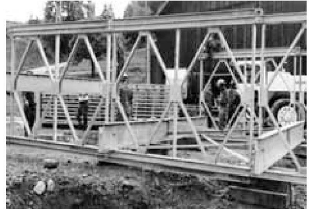
Costruzione di un ponte militare provvisorio Maby & Johnson in sostituzione del ponte distrutto dall'alluvione a Gross, Canton Svitto (2007).
