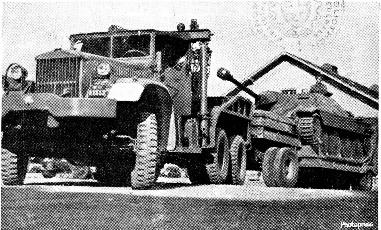
Cacciatore anticarro G 13 su rimorchio.
