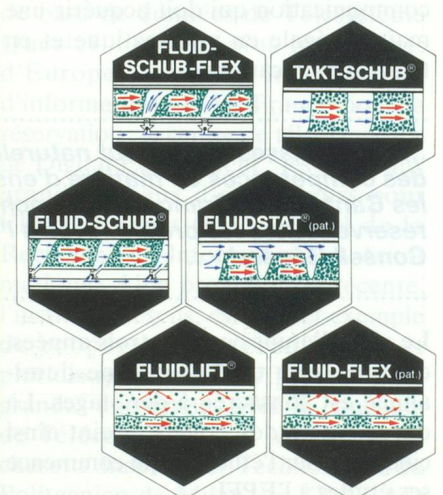
TRANSPORTS PNEUMATIQUES - PHASE DILUEE - VITESSE LENTE
