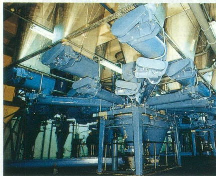
DOSAGE - PESAGE DANS UNE UNITE DE MELANGE POUR LE CAOUTCHOUC
