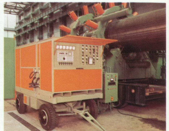
Installation moyenne fréquence mobile pour l'ajustement fretté de garnitures de rotors de turbogénérateurs.
