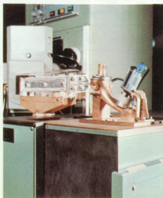
Générateur HF avec poste de brasage pour robinetterie en laiton.
