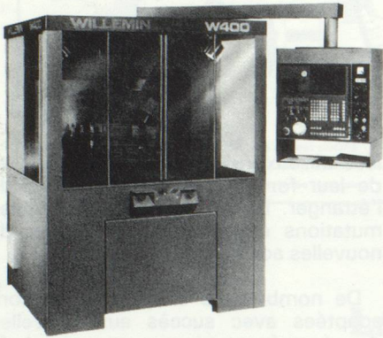
W-400 Centre d'usinage 5 axes, broche inclinable, magasin à 12, 24, 36 ou 48 outils, commande numérique NUM ou General Electric
