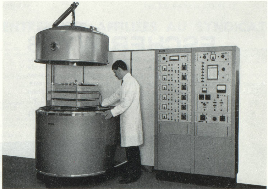
SUBLIMATEUR Type SM permettant le traitement de produits en ampoules, en flacons ou en vrac
