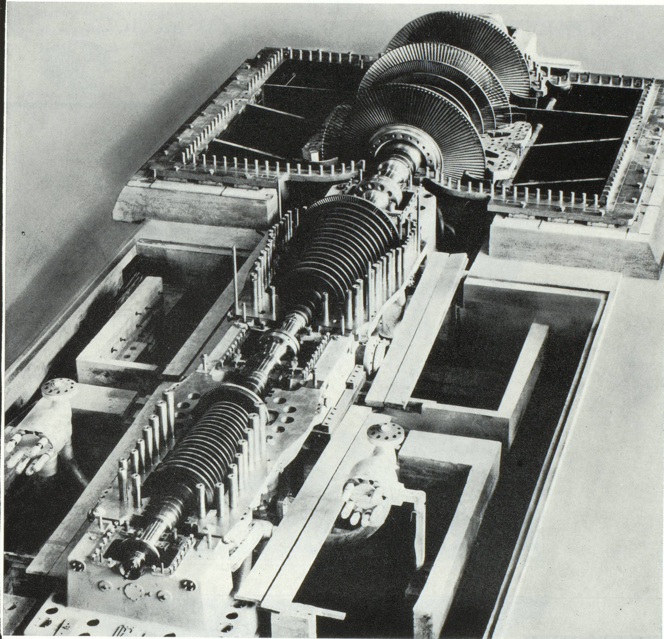
Turbo alternateur 150 MW Vouvry
