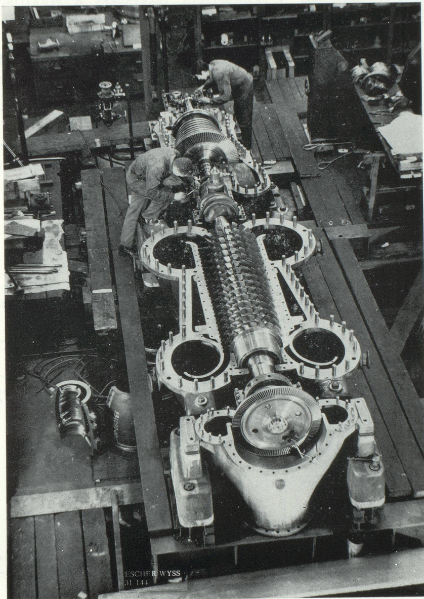
Turbo-groupe pour atelier d'acide nitrique.
