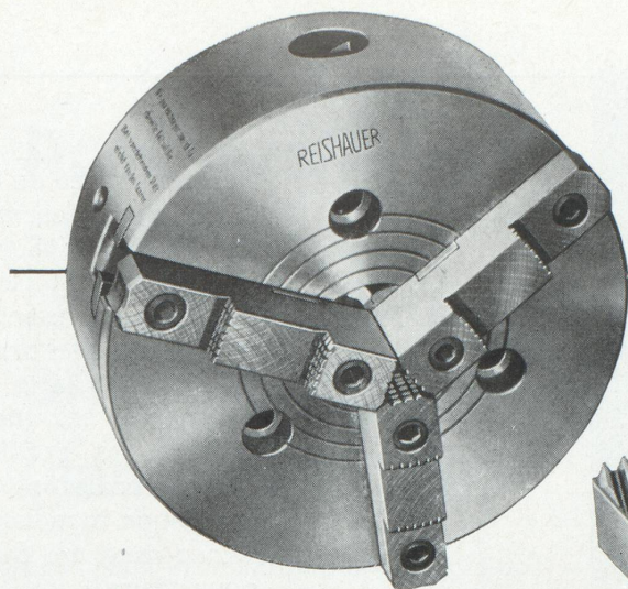
Mandrins de serrage à main avec denture rectifiée toutes faces
