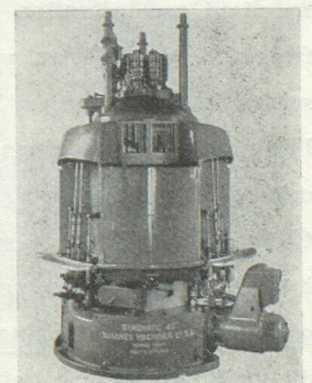
Tour automatique pour l'usinage en reprise.
