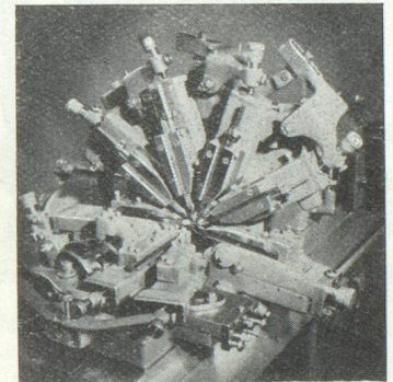
Les 6 outils radiaux d'un tour à décolleter.
