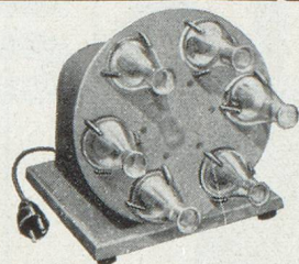
Appareil pour la détermination de la résistance globale. Particulièrement utilisable dans les laboratoires d'hématologie pour la résistance mécanique des éléments globulaires du sang. (Appareil électrique.)
