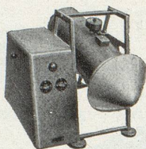
Fournaise électrique à bombe. Pour fonctionnement agité ou oscillé, régulation automatique de température jusqu'à 350° C.
