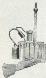
Micro-thermostat électrique. Adaptable sur tous les récipients appropriés. Grande précision et constance pour de longues durées d'utilisation. Agitation à hélice silencieuse.
