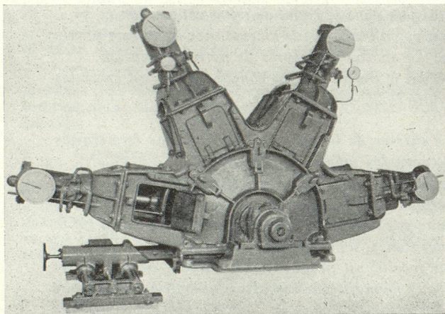
Défibreux à 4 presses pour le traitement du bois.
