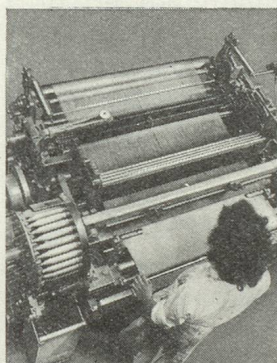
Notre couverture : Métier automatique moderne RUTI, à une navette du modèle BAN à bâti surbaissé
