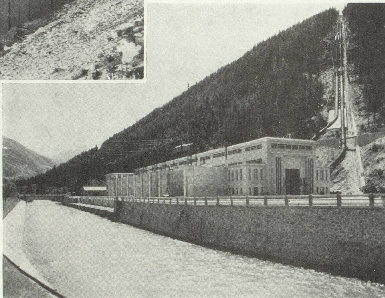
La centrale de Malgovert (Photo H. Baranger)
