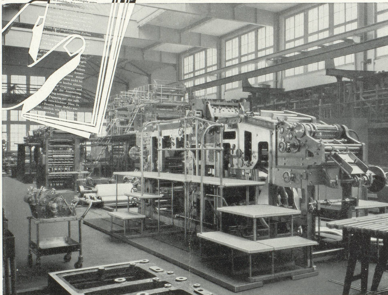
Vue partielle des halles de montage des rotatives WIFAG
