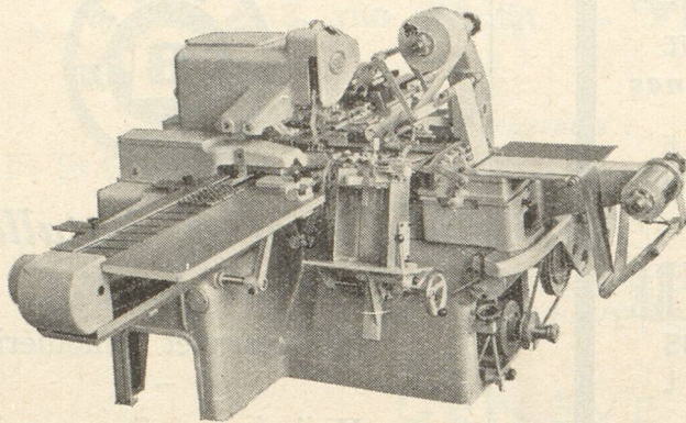
Empaqueuse pour tablettes de chocolat à grand rendement
