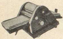
CENTO 25 — la machine qui imprime et organise sans encre et sans stencil
