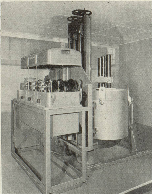
Four d'investigation de 60 kW muni de régulateurs Rex-Sécheron
