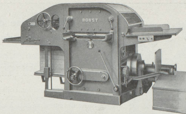
J. BOBST ET FILS S. A., PRILLY-LAUSANNE AUTOPLATINE marge à main : presse à platine automatique pour le découpage et le refoulement au moyen de « filets » (3.600 feuilles/h.).
