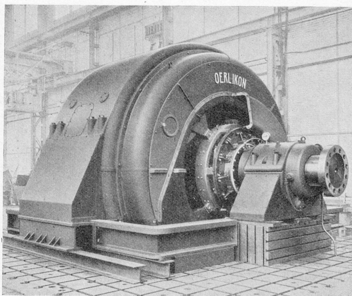
Fig. 1. — Alternateur de 37.500 K. V. A., vitesse 500 tours par minute pour la Centrale de la Dixence (Suisse)
