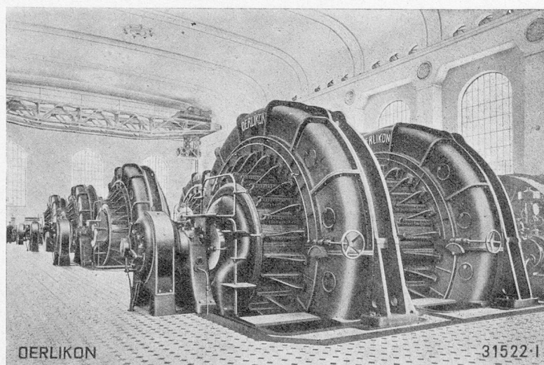
Fig. 6. — Génératrice à courant continu, 12.000 kW., usine de Rjukanfos (Norvège)
