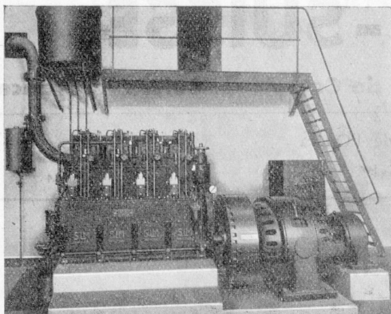
Projecteurs Marchal à Pantin Groupe électrogène à huile lourde 130 kwts
