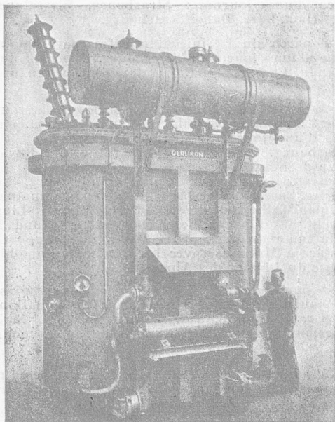
TRANSFORMATEUR POUR EXTÉRIEURS 3000 KVA 11500/23500 VDT9 AVEC CONSERVATEUR ET RÉFRIGÉRANT
