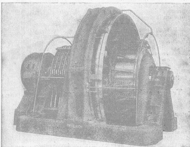
COMMUTATEUR 5.000 KW, 10 000 AMPÈRES
