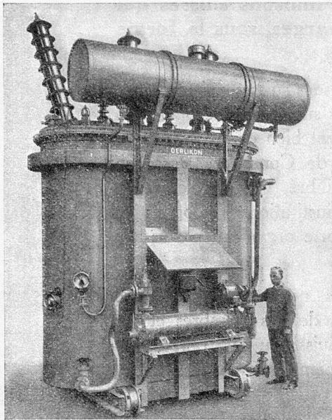
TRANSFORMATEUR 3000 KVA AVEC RÉFRIGÉRANT
