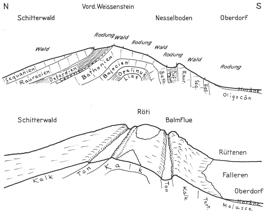
Abb. 1. Wald und Rodung im Weissensteingebiet (Geologie nach A. Buxtorf und P. Staehelin)
