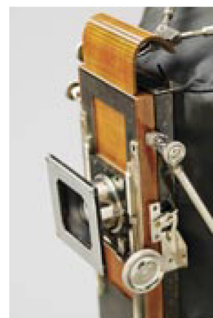
Fotocamera di Albrecht Meydenbauer, dettaglio con obiettivo, 1898
