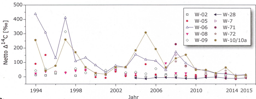
Figur 12: Zeitreihe der Netto \Delta^{14}\text{C} -Werte westlich des Rheins (östlich der KVA). Am Standort W-28 wird die ^{14}\text{C} unbelastete Stadtluft gemessen. Liegen von einem Standort mehrere Messungen vor, so ist der höchste Netto \Delta^{14}\text{C} -Wert eingetragen.
