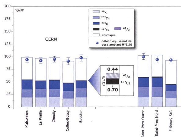
Figure 3: Contributions individuelles au débit d'exposition ambiante déterminées par spectrométrie gamma in situ pour les sites voisins du CERN examinés en 2011, et comparaison avec les résultats obtenus à St-Prex/VD ainsi qu'à Fribourg.
