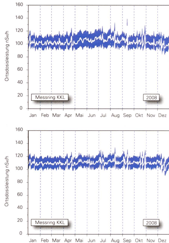
Figur 6: Wertebereiche aus Tagesmittelwerten für die Messringe KKL, KKM.
