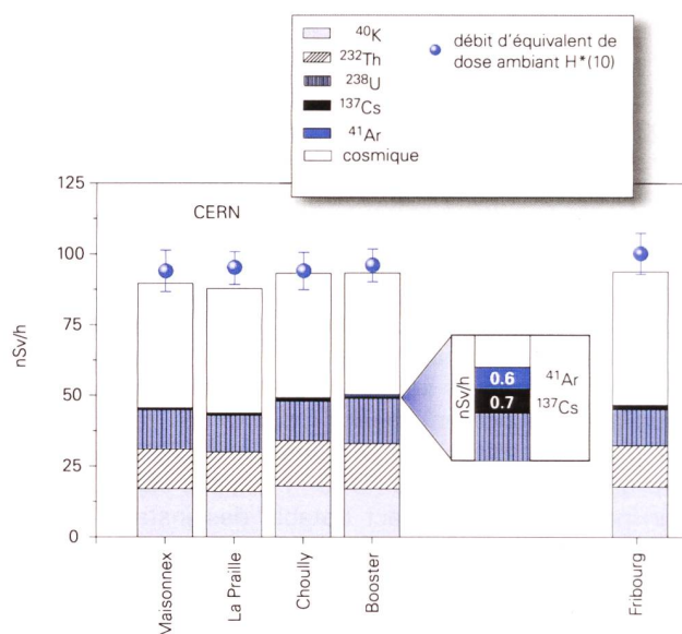
Figure 3: Contributions individuelles au débit d'exposition ambiante déterminées par spectrométrie gamma in situ pour les sites voisins du CERN examinés en 2008, et comparaison avec les résultats obtenus à Fribourg.
