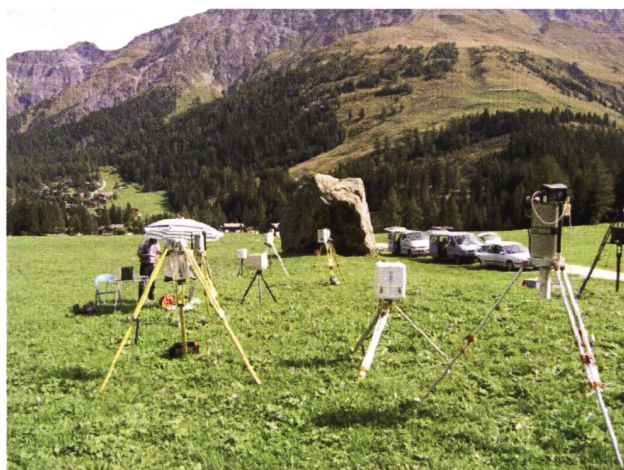
Figure 4: Instrumentation in situ des différents participants sur le site de mesure de La Fouly.
