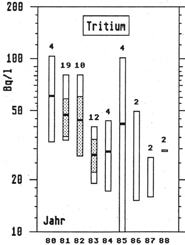
Fig.5.13.a: ARA Teufen
