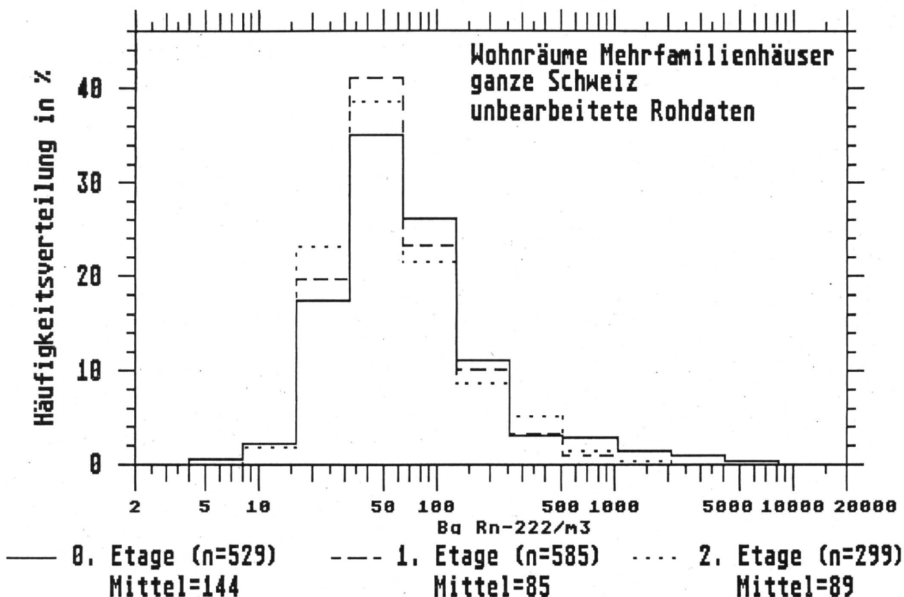
Fig.2.2.b: Radonmesswerte bis inkl. Winter 88/89
