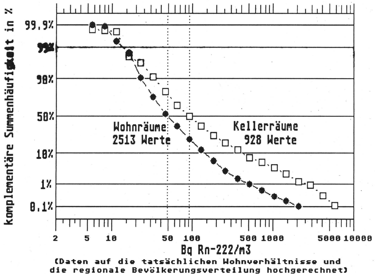
Fig.2.7: Radon-Konzentrationen in Schweizer Häusern bis incl. Winter 88/89
