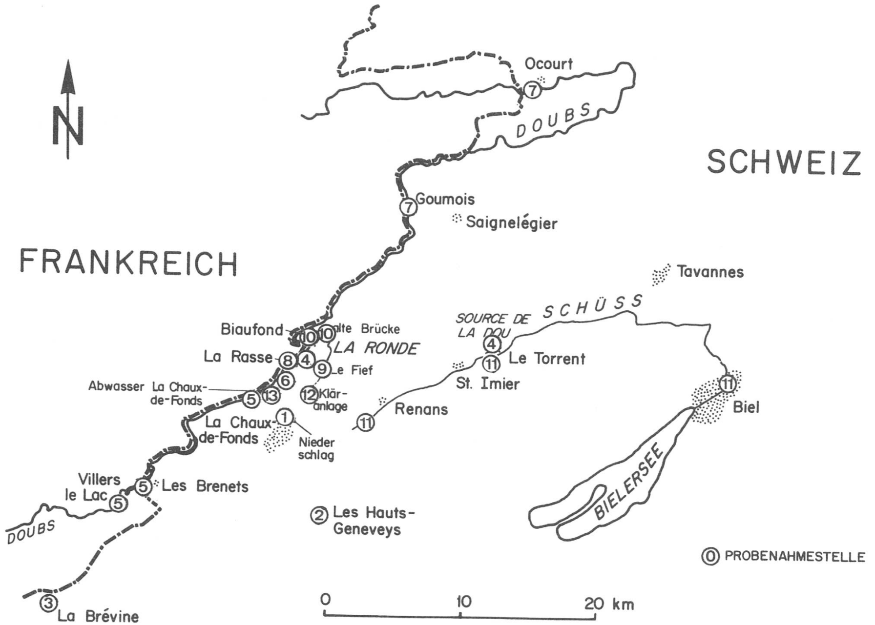
Fig. 16. Probenahmestellen für Tritium in Wasser im Raum La Chaux-de-Fonds, Zahlen vgl. Tab. 9 (EAWAG)
