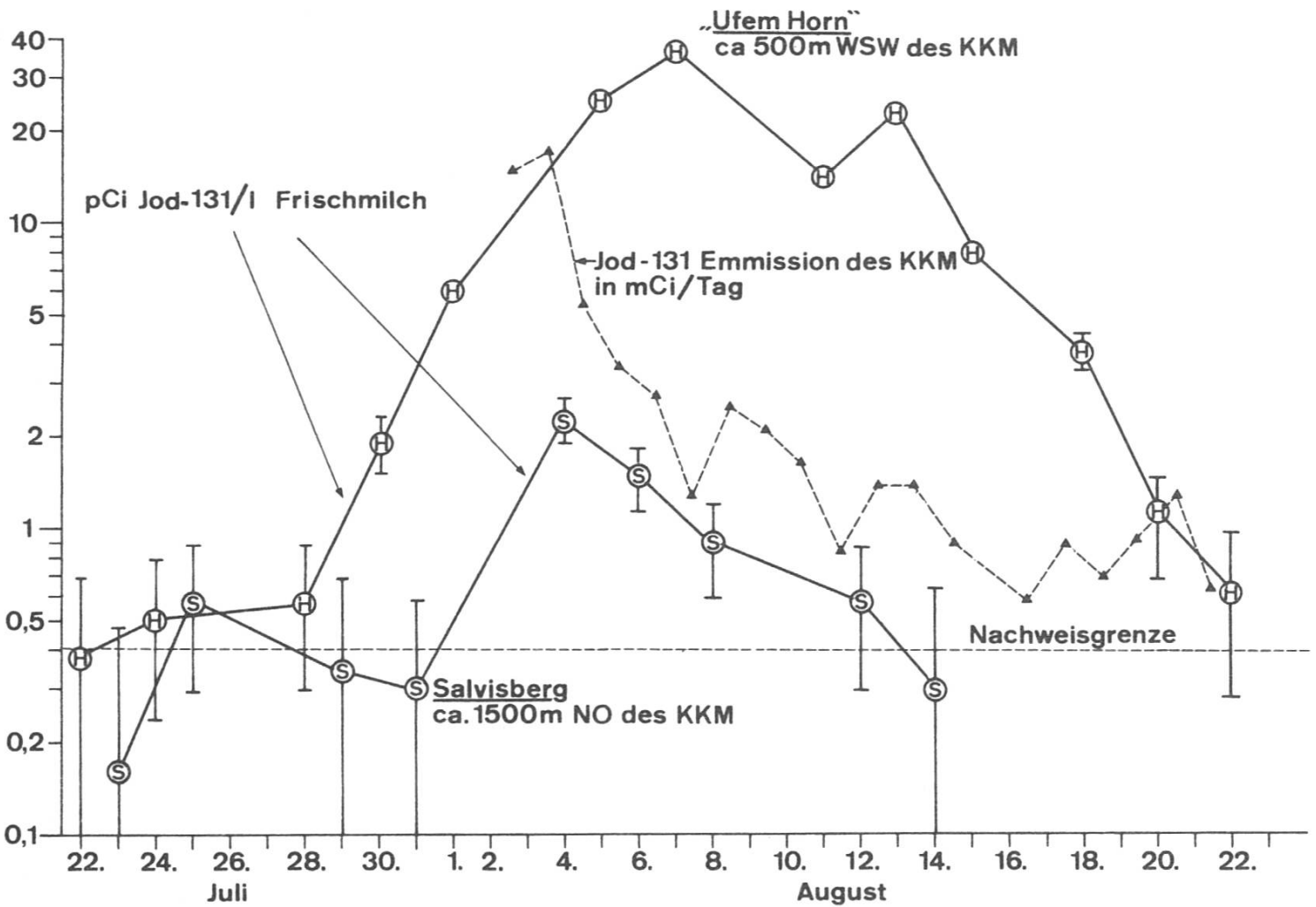
Fig. 9. Jod-131-Emission aus dem Kernkraftwerk Mühleberg und Jod-131-Gehalt in der Milch von ausgewählten Stellen in den Haupt-Windrichtungen, Juli/August 1975 (Genauigkeit an der Nachweisgrenze: \pm 50\% bei einfacher Standardabweichung) (FR) Emission d'iode-131 par la centrale nucléaire de Mühleberg et teneur en iode-131 de lait provenant d'endroits choisis dans les directions principales du vent, juillet/aout 1975 (Précision à la limite de détection: \pm 50\% au niveau de confiance de 68%) (FR)
