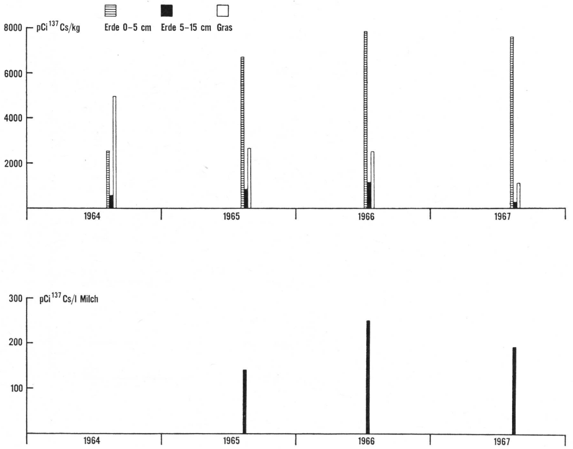
Fig. 15. Cs-137-Aktivität von Erdboden, Gras und Milch, Davos-Dischmatal/GR, 1964-1967. Fig. 15. Activité en Cs-137 du sol, de l'herbe et du lait à Davos-Dischmatal/GR, 1964-1967.
