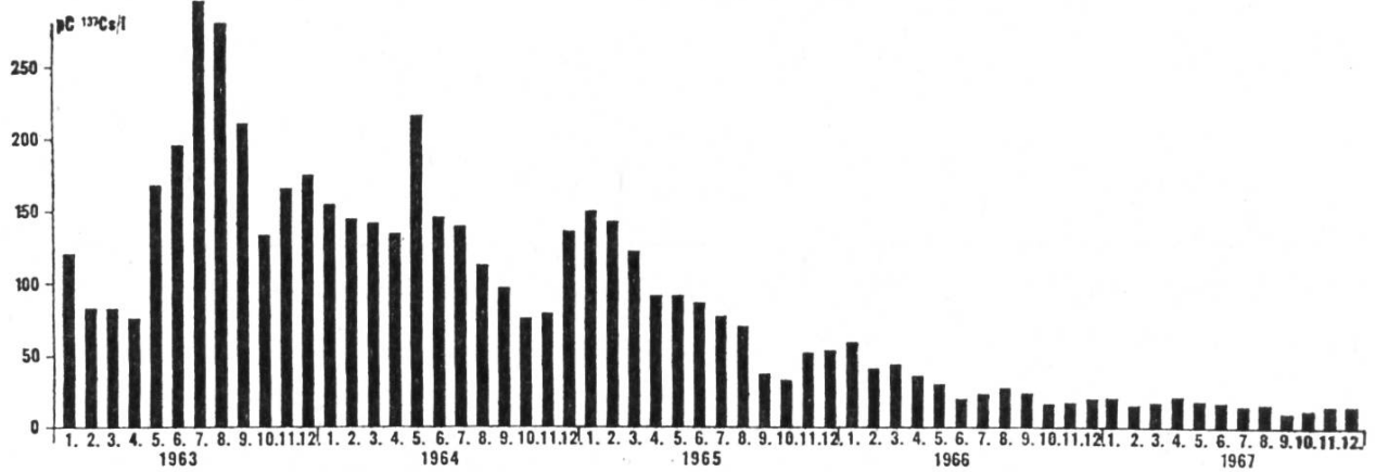
Fig. 13. Oben: Cs-137-Gehalt von Viehfutter (monatliche Probenahme), Ostschweiz 1963–1967. Unten: Cs-137-Gehalt von Milch (monatliche Probenahme zwei Tage nach derjenigen des Futters), Ostschweiz 1963–1967.
