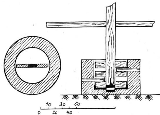
Teigknetmaschine
