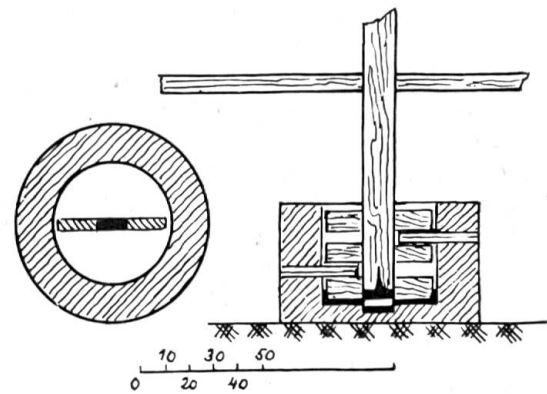
Teigknetmaschine
