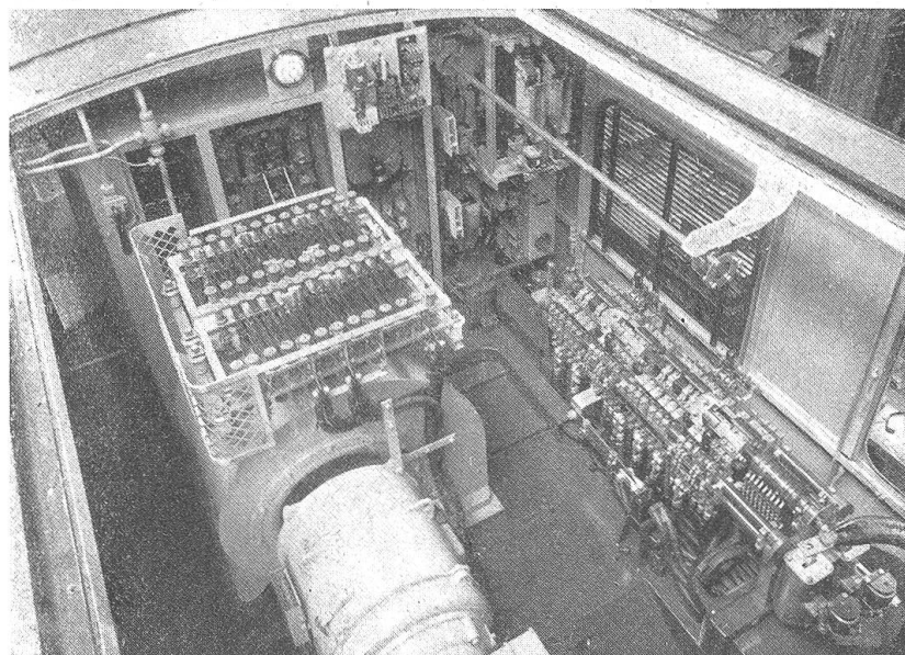
Abb. 17. Maschinenraum einer modernen Lokomotive mit den komplizierten Schaltapparaten
