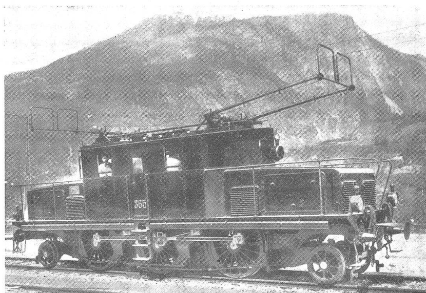
Abb. 6. Diese Drehstromlokomotive hat während der Jahre 1906 bis 1930 die Züge durch den Simplontunnel befördert. Leistung 1100 PS, Maximalgeschwindigkeit 70 km pro Stunde
