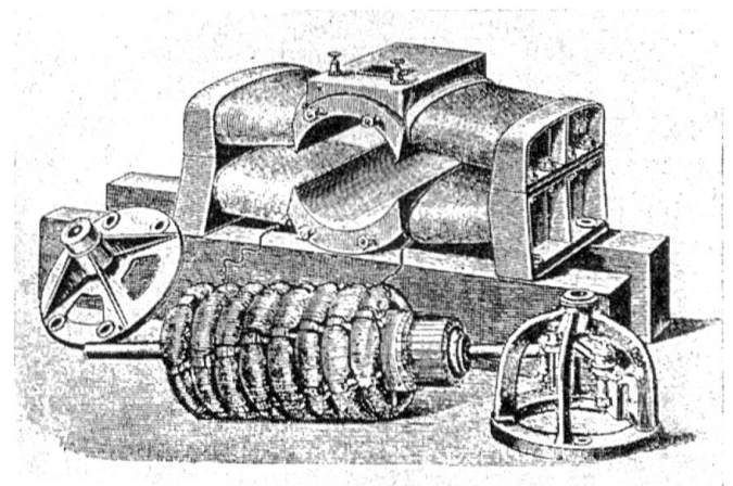
Abb. 1. Erster schweizerischer Gleichstromdynamo für Maschinenbetrieb (Baujahr 1875). Erbauer: Emil Bürgin (Reproduktion aus: „Wyssling, die Entwicklung der schweizerischen Elektrizitätswerke in den ersten 50 Jahren.“ Herausgeber: Schweizerischer Elektrotechnischer Verein)
