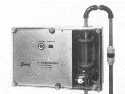
Probeentnahmegerät PE 76.
