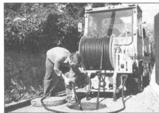
Mit Kanalreinigungsgerät
