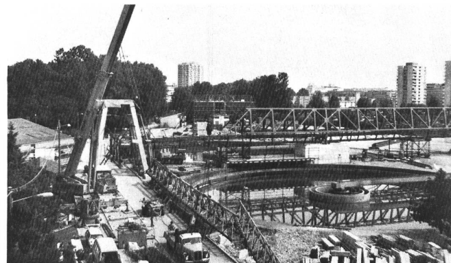
Im Vordergrund eines der beiden bestehenden Vorklärbecken, in der Bildmitte ein Teil der Stahlkonstruktion des Energiekanals und im Hintergrund das neue Rechengebäude.
