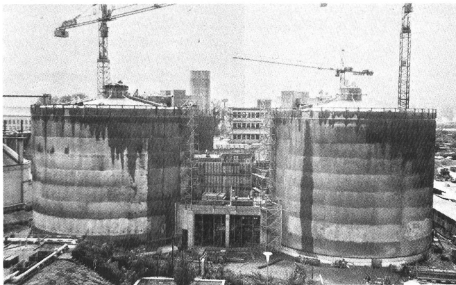
Zwei der vier neuen Schlammbehälter für die Vorfaulung. Dazwischen das Dienstgebäude mit der Schlammpasteurisierung im Bau.
