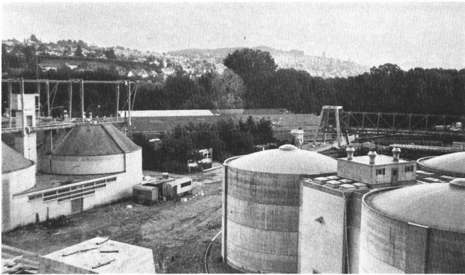
Links die Behälter der bestehenden Faulanlage, rechts davon die Behälter der Voreindickieranlage. In der Bildmitte das Dach der neuen Fahrzeugeinstellhalle und ein Teil der Stahlkonstruktion des rund 1 km langen Energiekanals, der über die gesamte Anlage führt.
