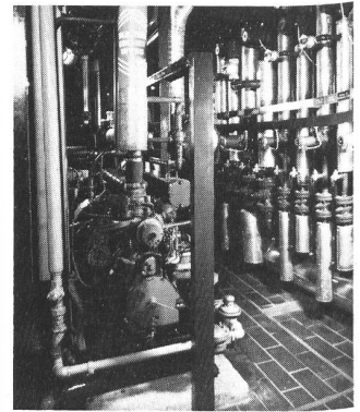
Gaswärmepumpenanlage zur Wärmegewinnung aus dem Hafenbecken.
